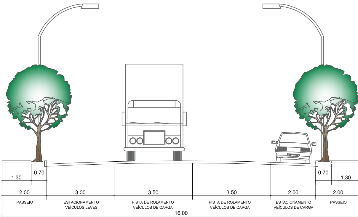
VIA COLETORA PRINCIPAL E VIA COLETORA SECUNDÁRIA
